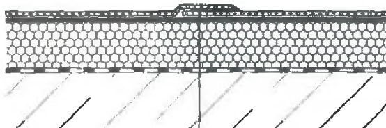
Příklad použití textilie FILTEK V při realizaci ploché střešy s fóliovou hydroizolací a tepelnou izolací z pěnového polystyrenu
