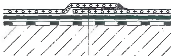
Příklad použití textilie FILTEK V při rekonstrukci ploché střešy s asfaltovou hydroizolací
