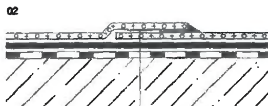
02 Příklad použití textilie FILTEK V při rekonstrukci ploché střechy s asfaltovou hydroizolací
